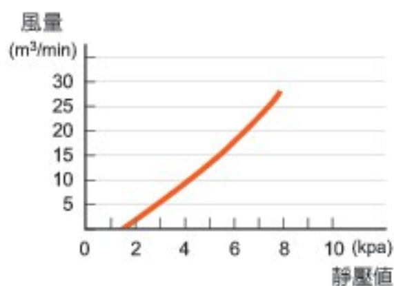
前濾心吸風量曲線圖
