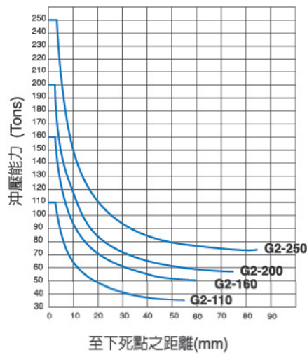
行程-能力曲線圖 (H)
