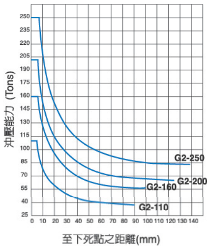
行程-能力曲線圖 (S)(V)
