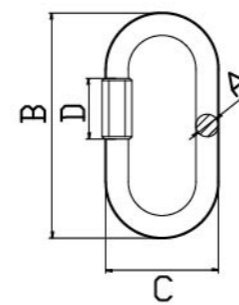
Quick Link LQ01
