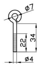
Bolt/Eyelet Stud Bolt-04
