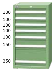
EA-10072 H1000xW566xD607 EB-10072 H1000xW718xD607 ED-10072 H1000xW718xD759
