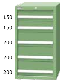
EA-10052 H1000xW566xD607 EB-10052 H1000xW718xD607 ED-10052 H1000xW718xD759
