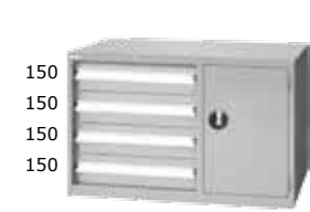
ELS-274 H700xW1000xD515 抽屜配置：150x4 第一層附分類盒，其餘每層皆附隔板二支
