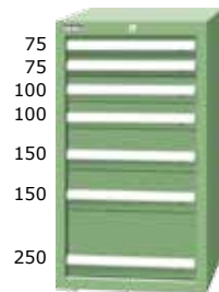
EA-10073 H1000xW566xD607 EB-10073 H1000xW718xD607 ED-10073 H1000xW718xD759
