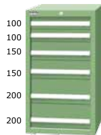
EA-10061 H1000xW566xD607 EB-10061 H1000xW718xD607 ED-10061 H1000xW718xD759
