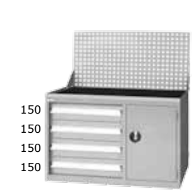
ELS-274A H1193xW1000xD515 抽屜配置：150x4 第一層附分類盒，其餘每層皆附隔板二支 產品內含：掛板組+上框(附膠墊) KPQ-B掛鉤一組 (12 pcs)
