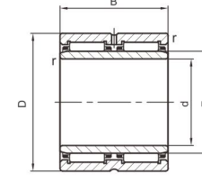
NA 69 (F≥40) double row
