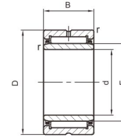
NKI ,NKIS, NA49 NA 59 ,NA 69(F≤35) single row
