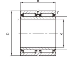
NA 69 (F≥40) double row
