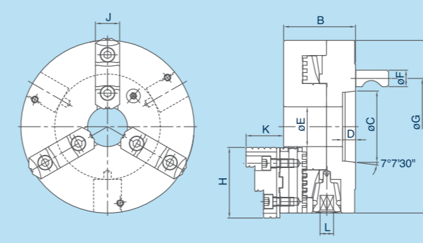
尺寸圖 > Dimensions
