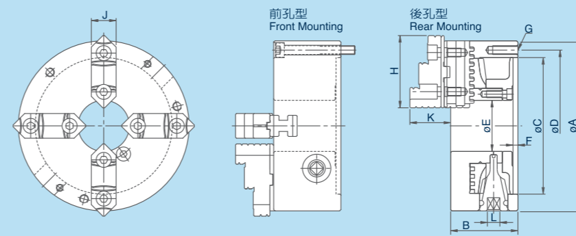
尺寸圖 > Dimensions
