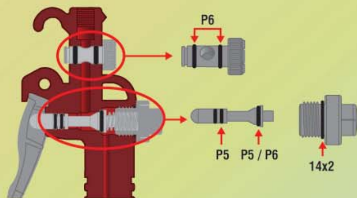
內部構造剖面圖 Sectional View
